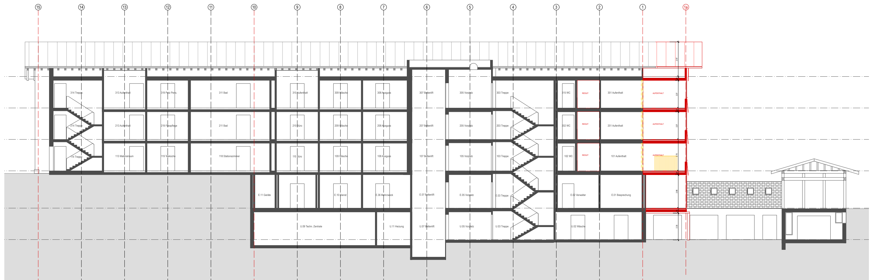
Längsschnitt
